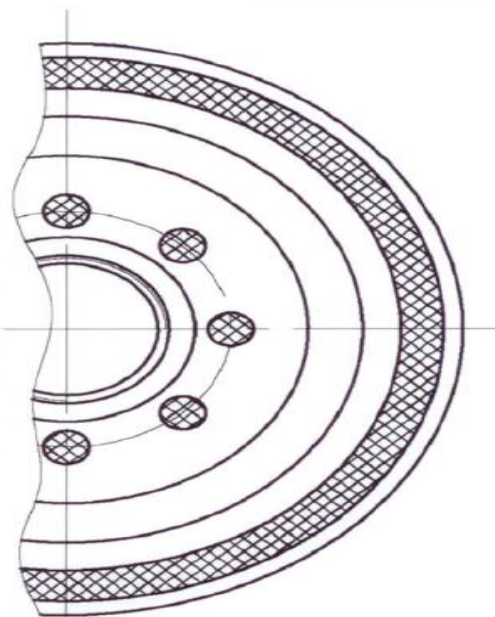
A向 1 : 1
